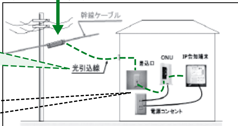
設置概要図（参考）
